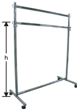
2 角バー2段ラック Size: W1200 × D550 × H1235 / H1475~2450 商品番号: WR1200
